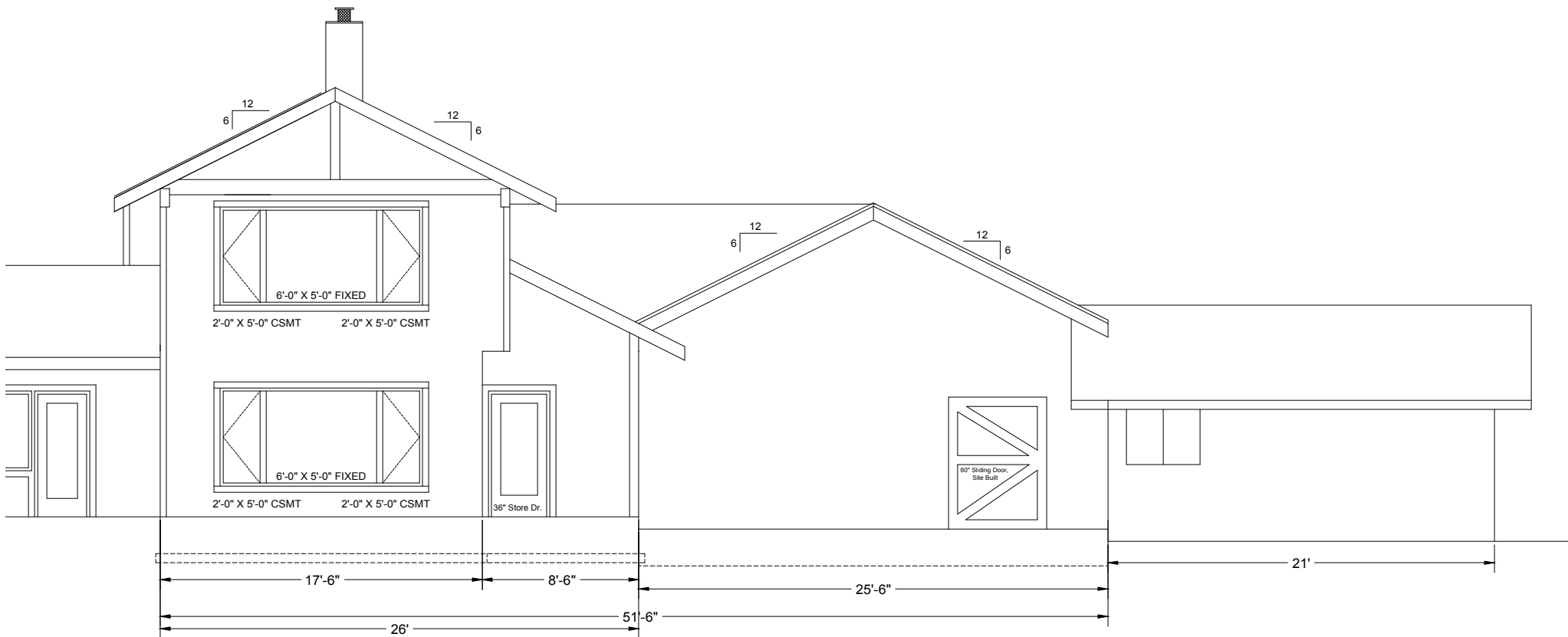
East Elevation Scale: 1/8" = 1'
